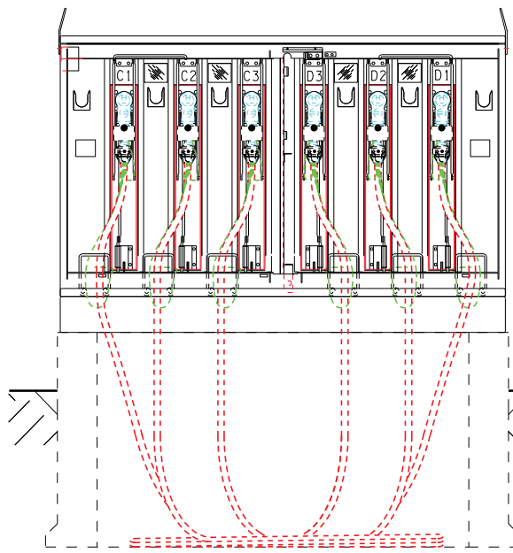
25T422DD*** (MSG-200-9) & 25T421DD*** (MSG-200-12) FUSE COMPARTMENT ( C & D )
