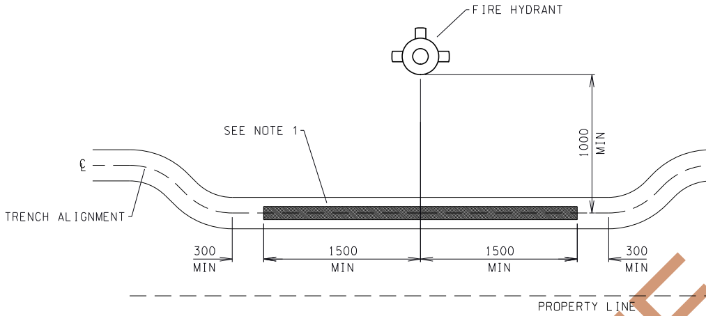
MECHANICAL PROTECTION PAST HYDRANT SCALE: N.T.S.
